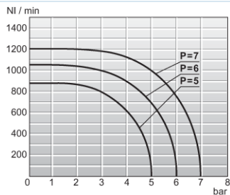
Flödesdiagramm 1/8"
