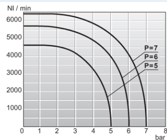
Flödesdiagramm 1/2"
