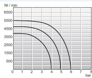
Doorstroombiagramma 1/2"
