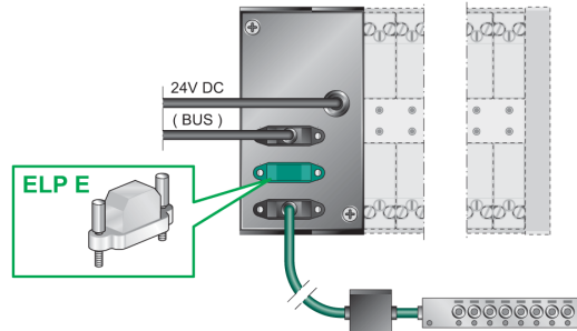
ELP I Päätytulppa INPUT PORT -liitântään
