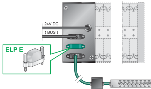
ELP E Päätytulppa EXTENSION PORT -liitântään
