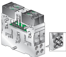
Moduuli magneettiventtiilisaarekkeelle sähköinen/sähköinen - _ _ -
