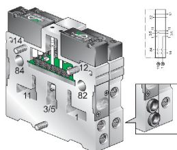
Moduuli Käyttöpaine-erotin - _ Y - yksittäisasemamoduulilla
