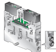
Enkelstationsmodul
