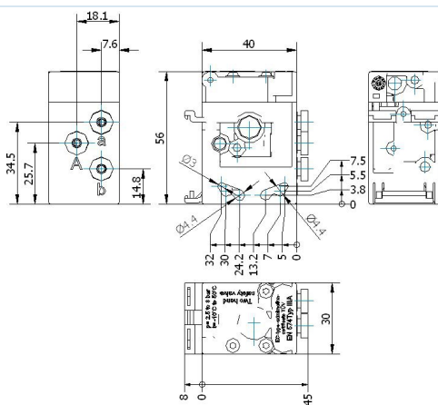
Rysunek wymiarowy
