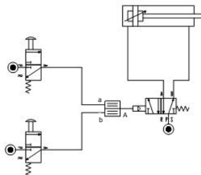
Schită de conectare
