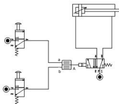
Anslutningsskiss
