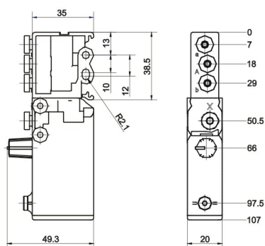
Rozměrový výkres
