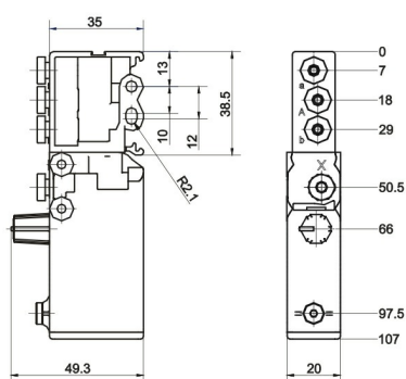
Dessin coté
