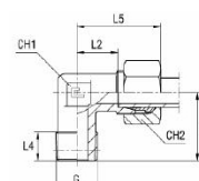
con anello tagliente B3
