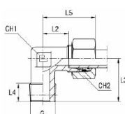
med B4-skärhylsa
