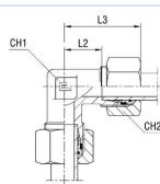
con anello tagliente B4
