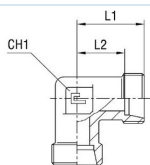
Grunnkropp
