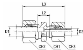
con anillo cortante B3
