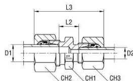
con anillo cortante B4
