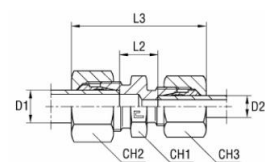
met B3-snijring
