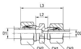
met B4-snijring
