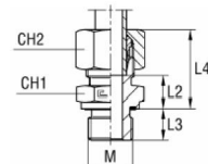
med B3-skärhylsa
