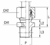
med B4-skæring
