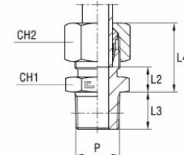
med B3-skæring
