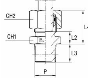
met B4-snijring
