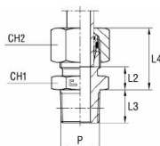
met B4-snijring
