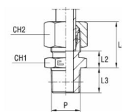
met B3-snijring
