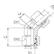
med B3-skärhylsa
