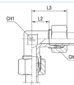
avec bague coupante B3
