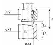
met B3-snijring
