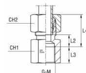
med B3-skärhylsa
