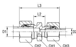
med B4-skæring
