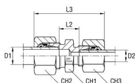
med B4-skärhylsa
