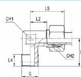
med B3-skæring
