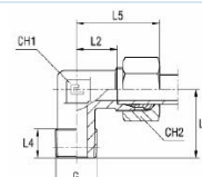
med B3-skærring
