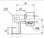
kanssa B3-leikkuurengas
