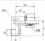
con anello tagliente B4
