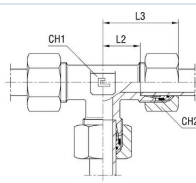
s řezným kroužkem B4
