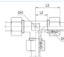
s řezným kroužkem B3
