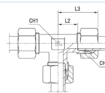
med B3-skärhylsa
