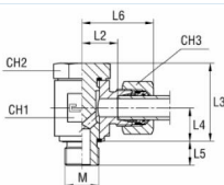
B4-leikkuurenkaalla
