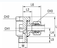
B3-leikkuurengasliittoksella
