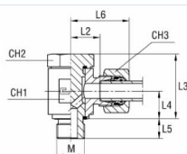
med B4-skärklämring
