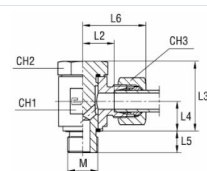
med B3-skärhylsa
