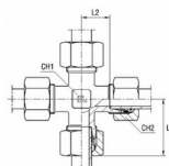
med B4-skärhylsa
