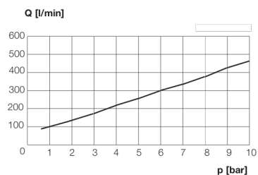
Gjennomstrømning
