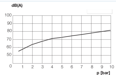
Støynivå
