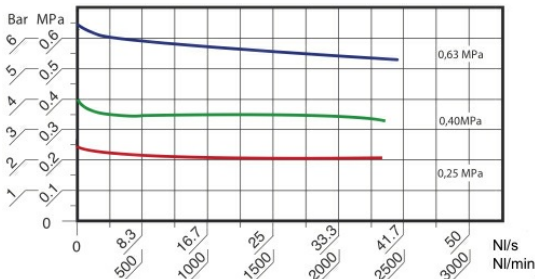
Presiune de intrare = 10bar, Debit volumic în condiții normale
