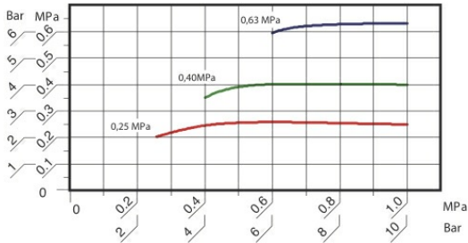
Debit constant = 750NI/min axă orizontală: Presiune de intrare axă verticală: Presiune de ieșire
