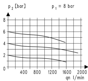
Virtauskaavio
