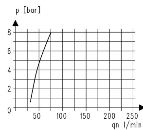
Öljysumuttimen toimintaraja
