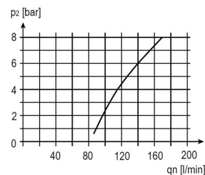
Olievernevelaar-inschakeldrempel
