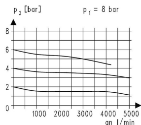
Doorstroombiagramma
