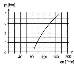
Olievernevelaar-inschakeldrempel
