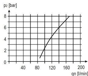
Öljysumuttimen toimintaraja
