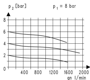
Virtauskaavio
