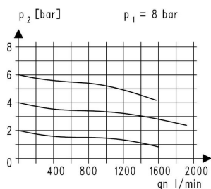
Strömungsdiagramm
