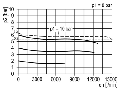
Virtauskaavio
