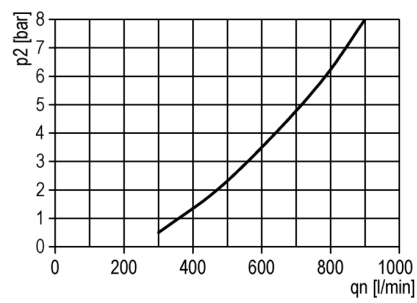
Olievernevelaar-inschakeldrempel
