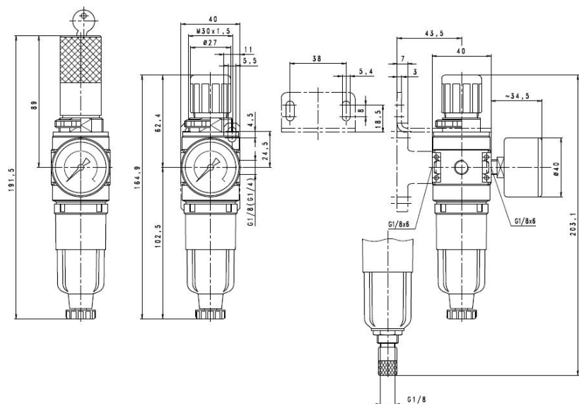
supapă de purjare semiautomată
