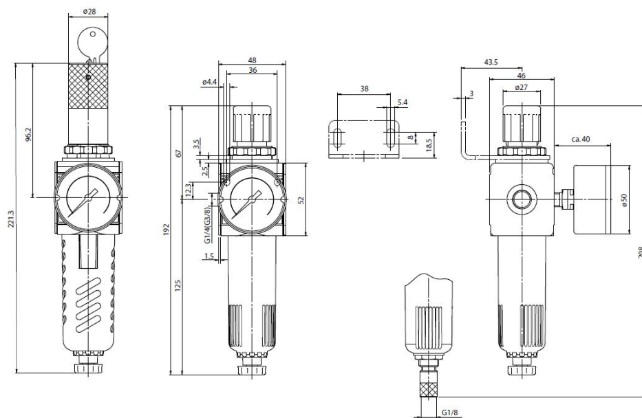
vanne de purge semi-automatique
