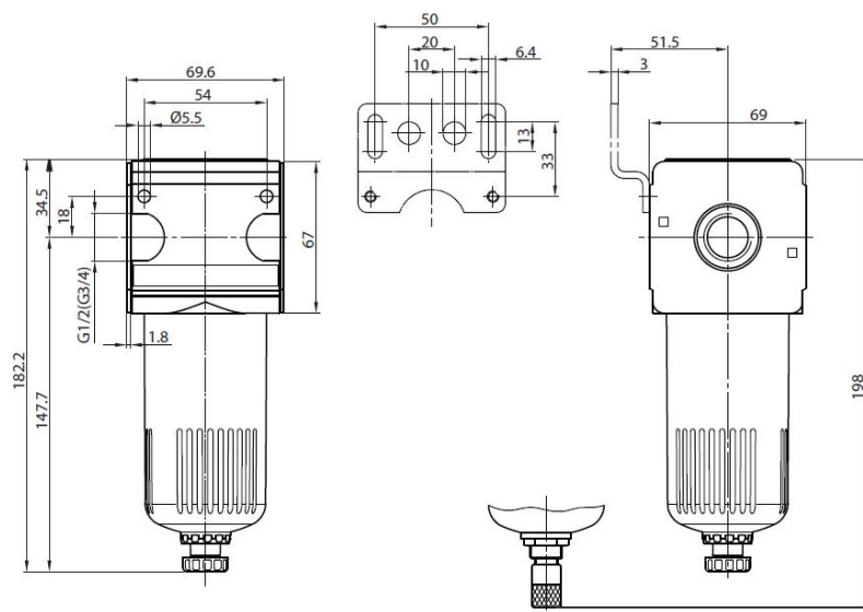
αυτόματη βαλβίδα αποστράγγισης
