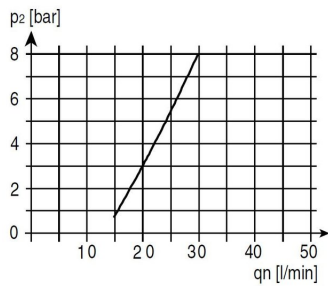
Umbral de respuesta del lubricador
