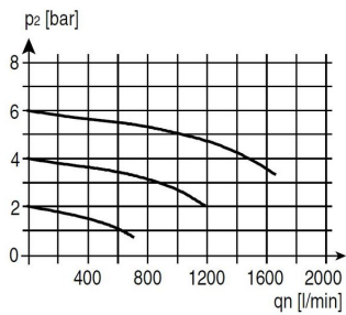
Diagrama de caudal
