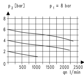
Průtokový diagramm
