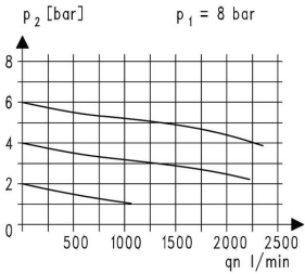
Strømningsdiagramm
