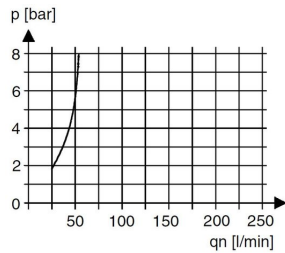
Olieforstøverens aktiveringsgrænse
