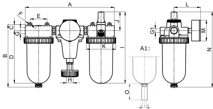
A1: automatisk aftapningsventil
