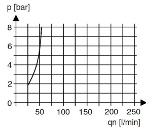
Olieforstøverens aktiveringsgrænse
